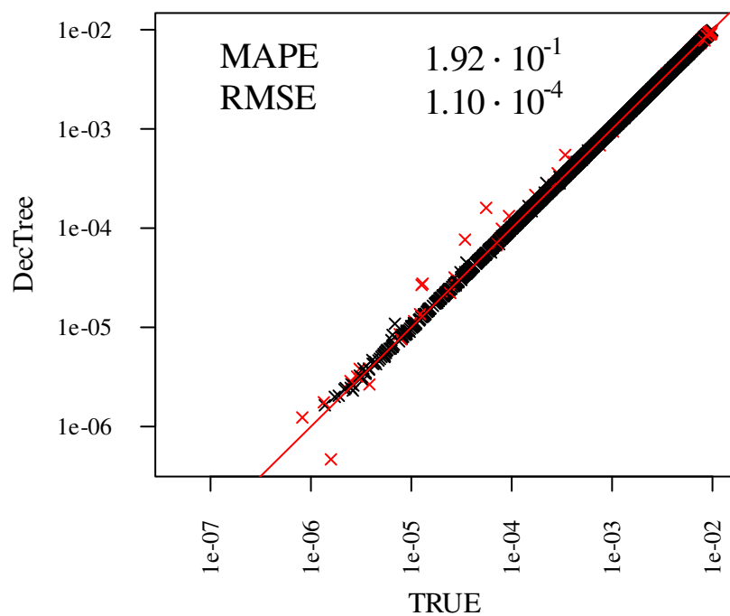
Metaschoepite
