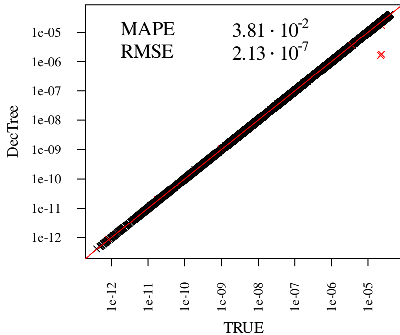
Metaschoepite
