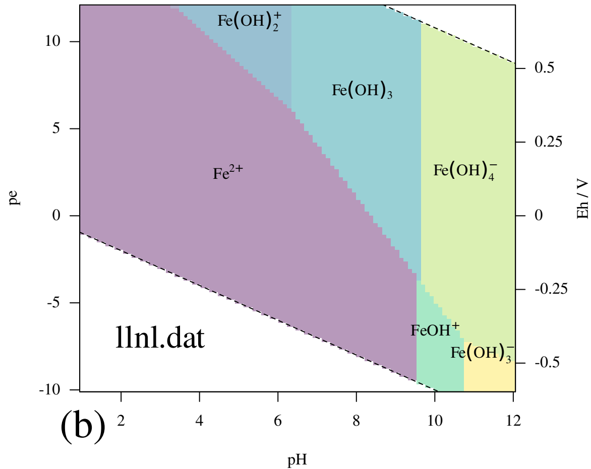
Pourbaix diagram for Fe T= 25 °C / P= 1 atm
