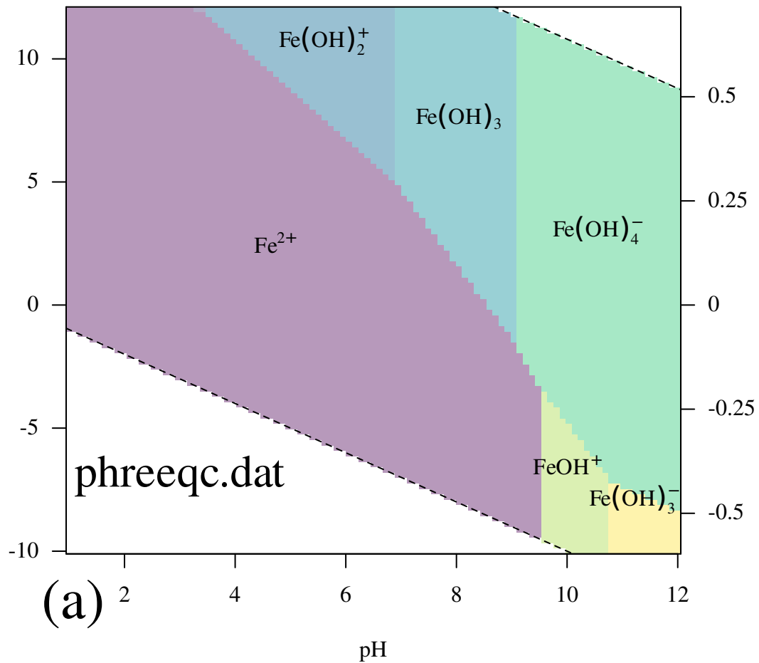
Pourbaix diagram for Fe T= 25 °C / P= 1 atm
